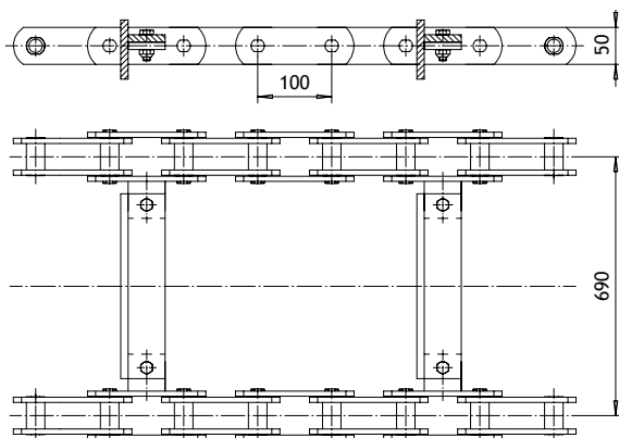
Matarkedja
