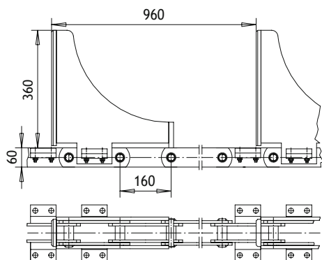
Timmerelevator
